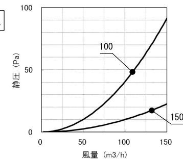
吸気
